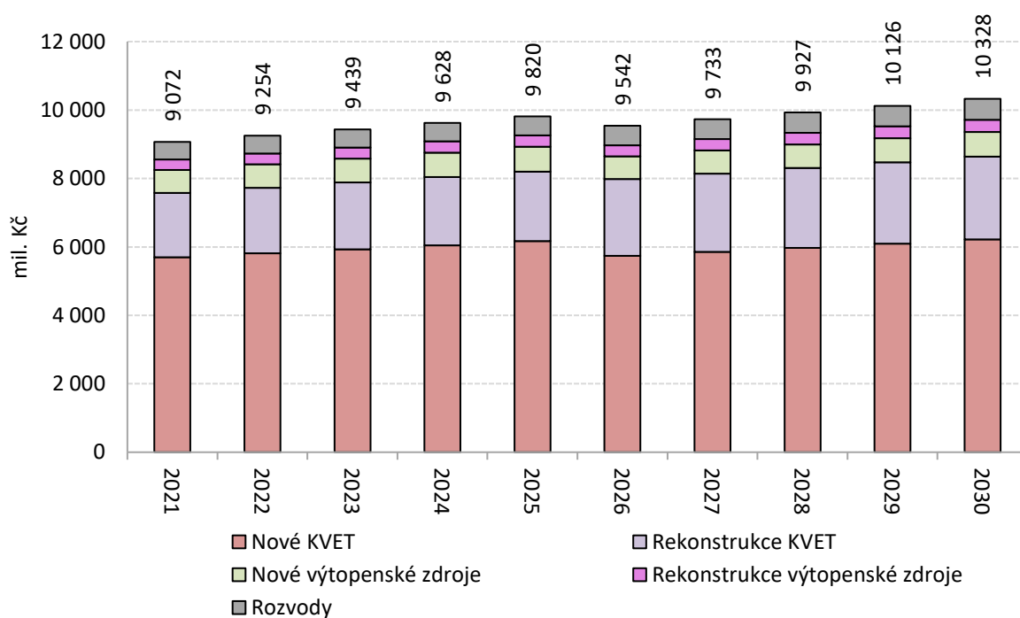
Graf č. 11: Rozložení nákladů na modernizaci teplárenství v letech v cenách běžného roku dle typu zdrojů a akce, optimistický scénář, běžné ceny daného roku (v mil. Kč)
