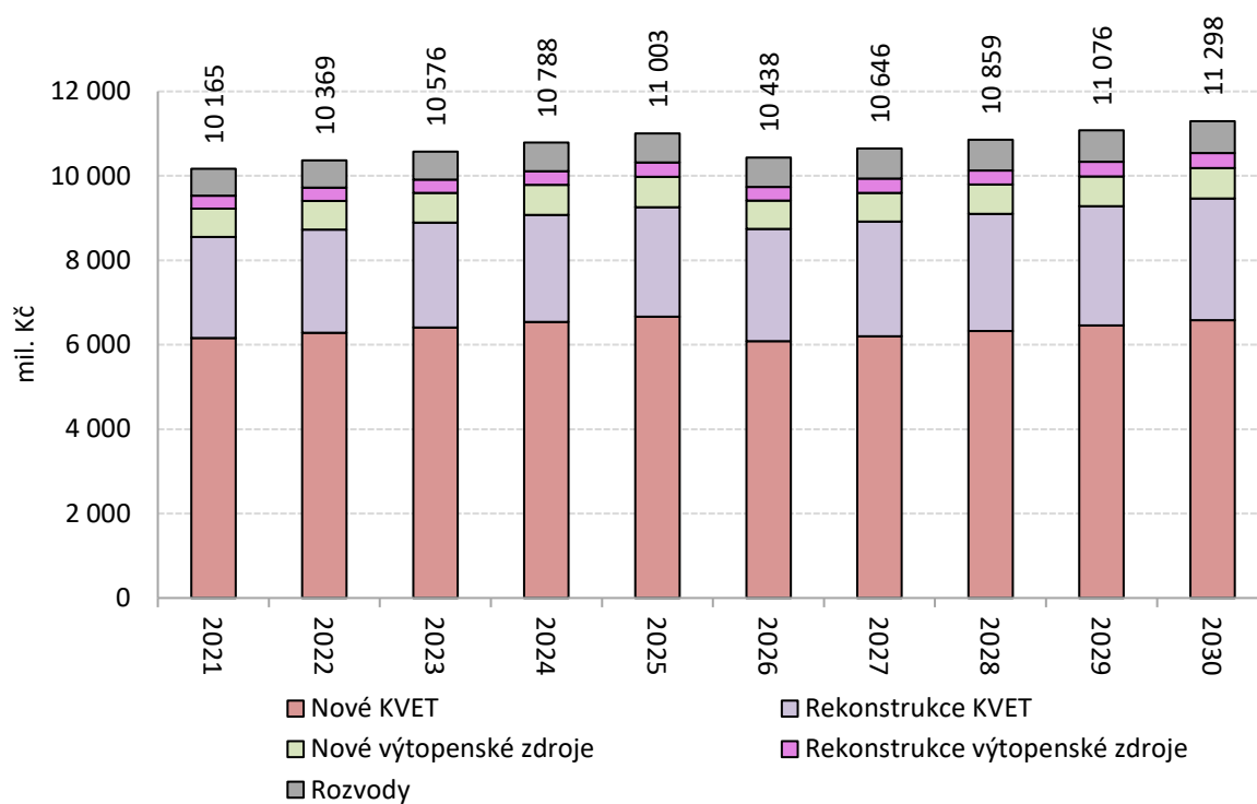
Graf č. 10: Rozložení nákladů na modernizace teplárenství v letech v cenách běžného roku dle typu zdrojů a akce, běžné ceny daného roku, konzervativní scénář (v mil. Kč)
